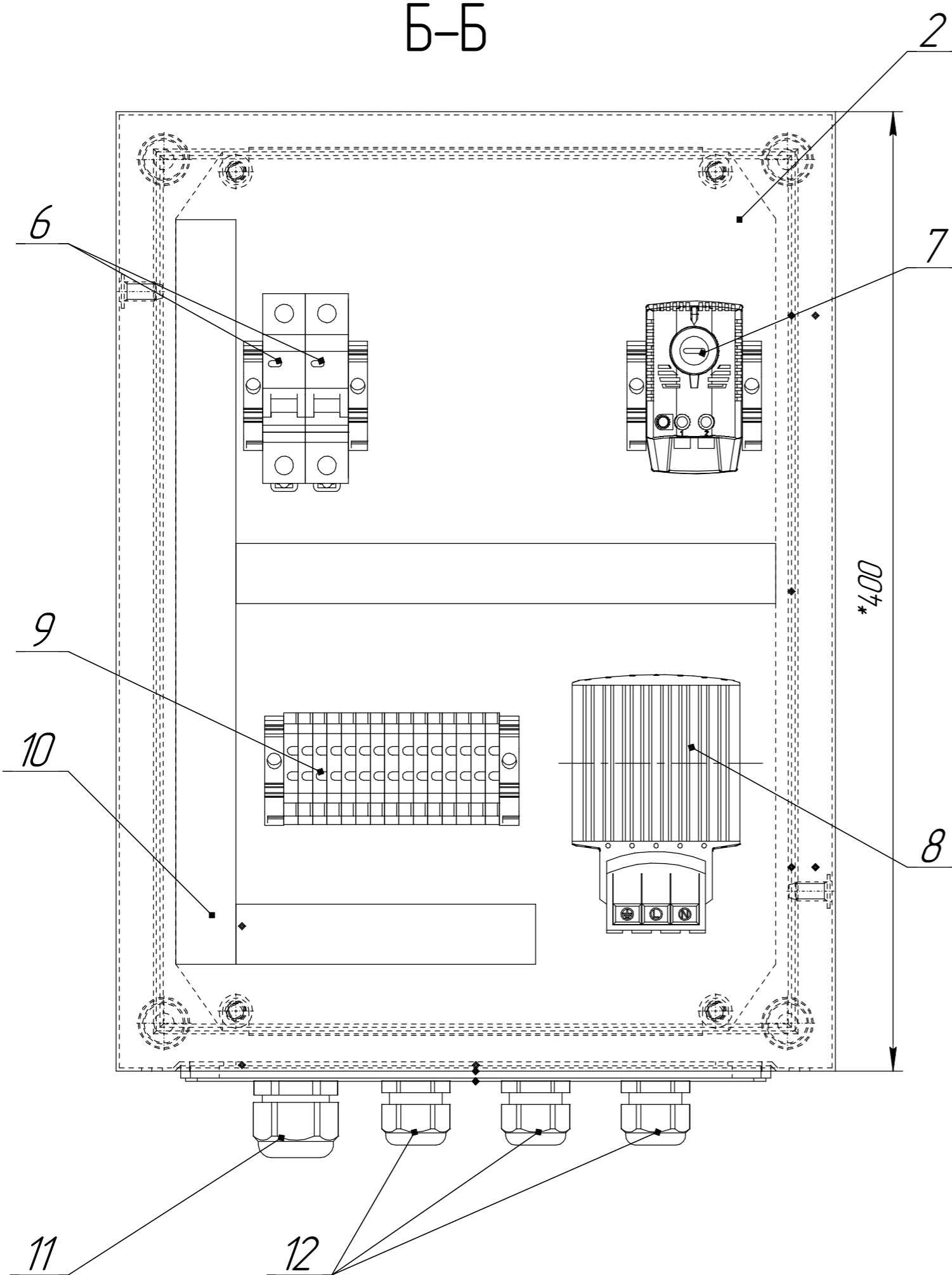
Вид в розрізі на монтажну панель без дверей
