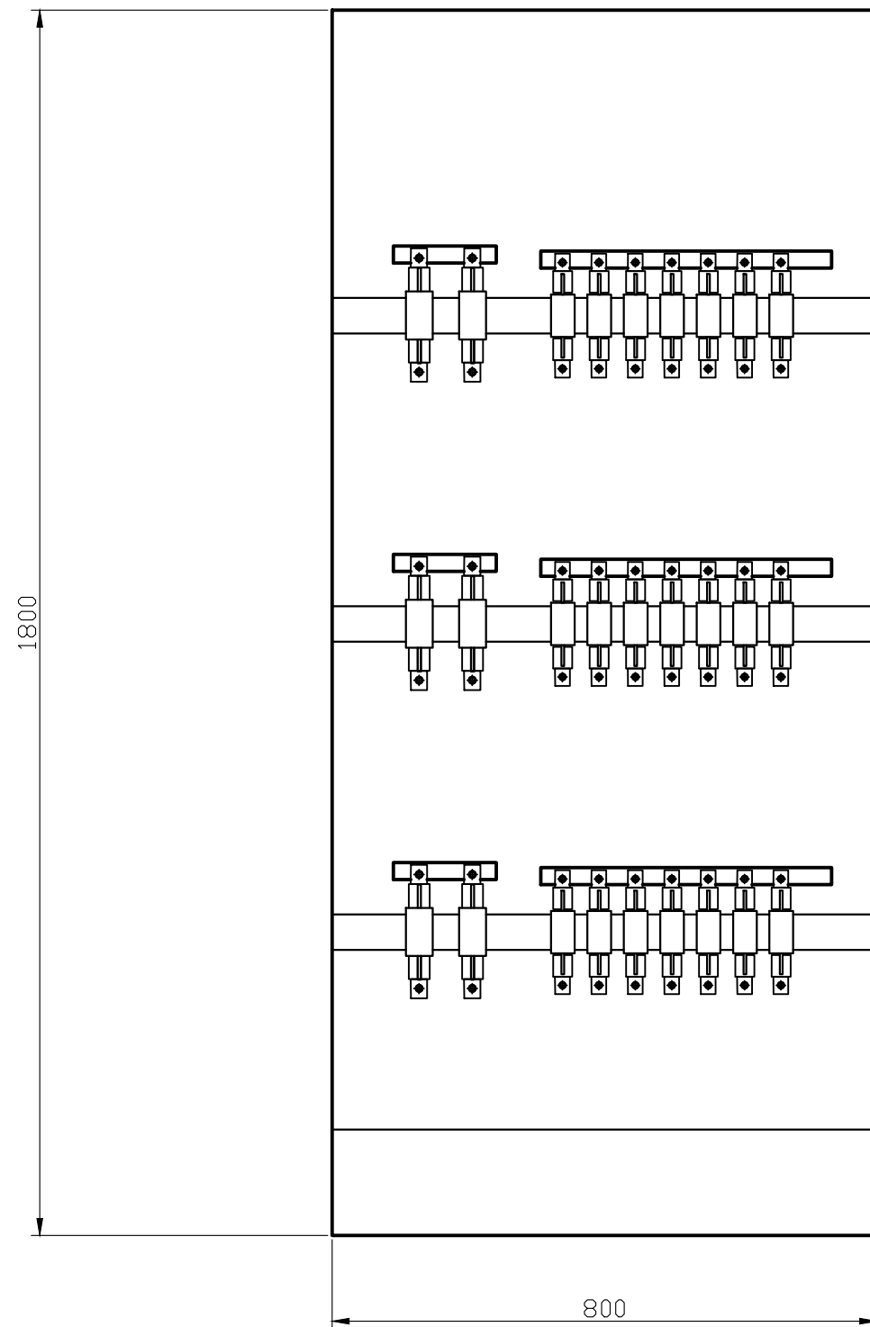
Вид спереду (двері не показані)
