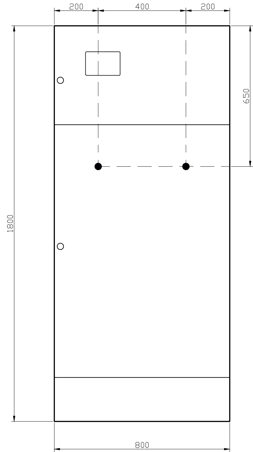
Вид спереду (двері шафи)
