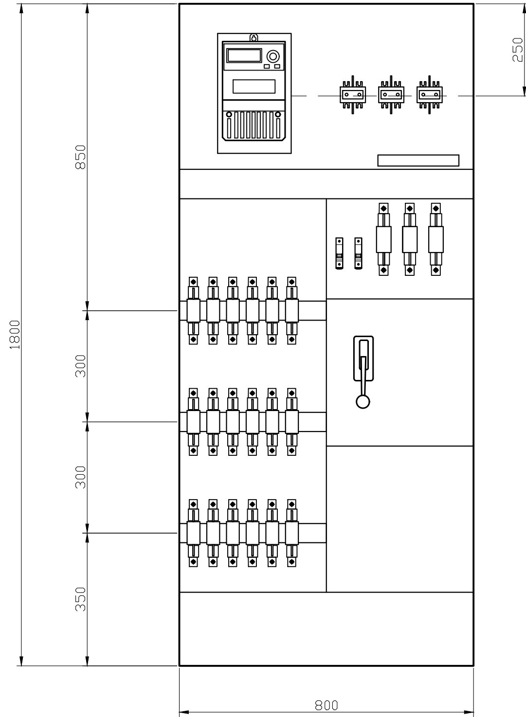
Вид спереду (двері не показані)
