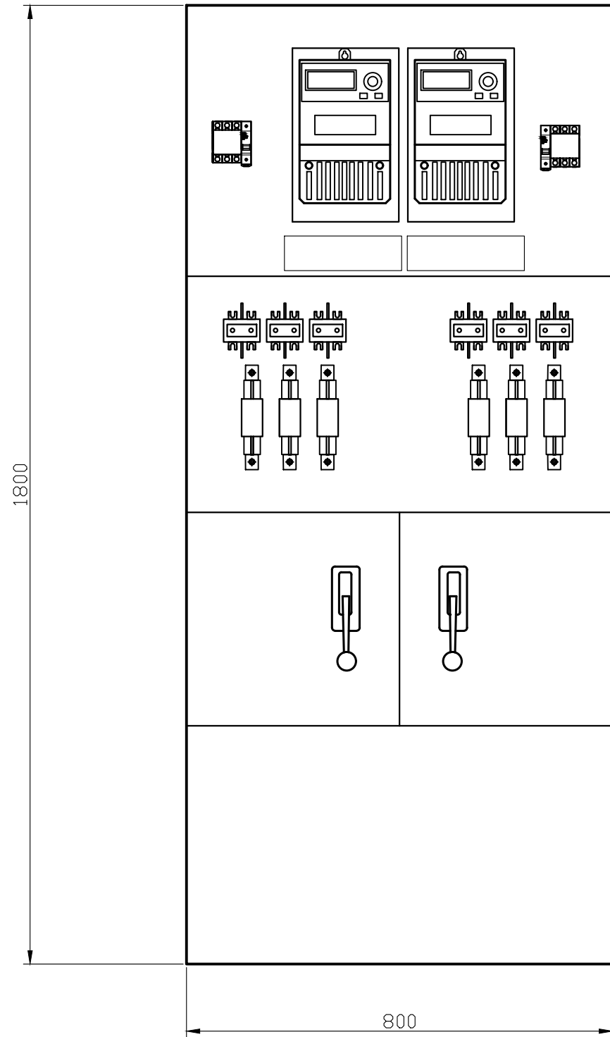
Вид спереду (двері не показані)
