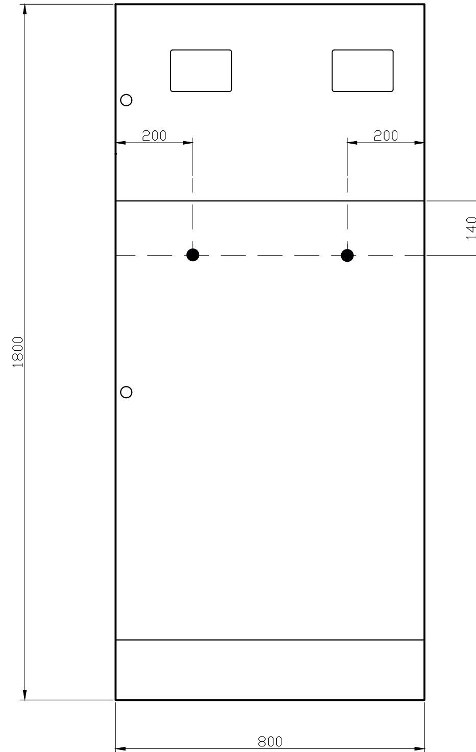
Вигляд спереду (двері шафи)
